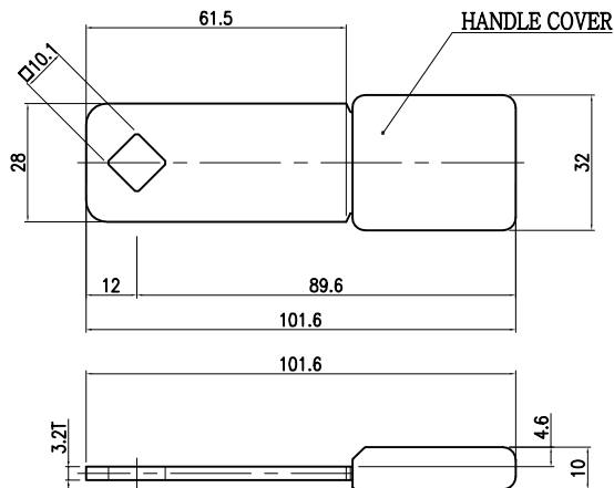
KA-110(SCP)
