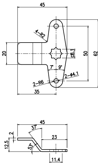
Rod Bar System 봉타입용(SCP)
